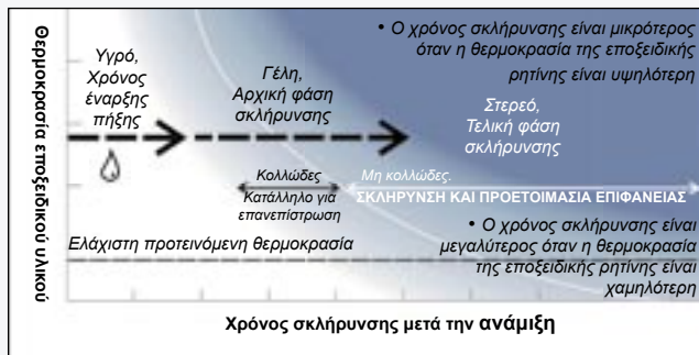
Σχήμα 1 Καθώς σκληρύνεται, το εποξειδικό μίγμα περνά από την υγρή φάση, μέσω του σχηματισμού γέλης (“gel”) τελικά σε στερεή κατάσταση.
