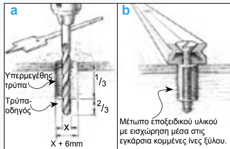
Σχήμα 16 Διανοίξτε υπερμεγέθεις τρύπες για να αυξήσετε την εκτεθειμένη επιφάνεια υποστρώματος και την ποσότητα εποξειδικού μίγματος γύρω από τη βίδα.
